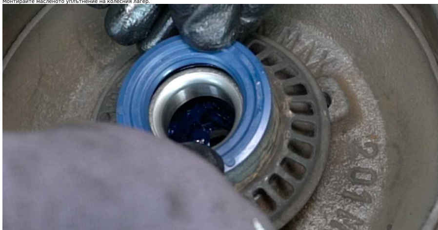
23 Обработете оста на главината. Използвайте универсален почистващ спрей. Използвайте грес за лагери.
