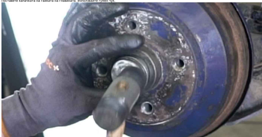
35 Обработете повърхността, където джантата прави контакт със спирания барабан. Използвайте керамична грес.
