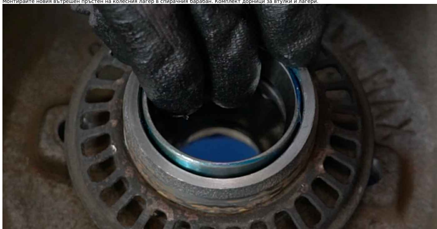
20 Обработете лагера на главината. Използвайте грес за лагери.
